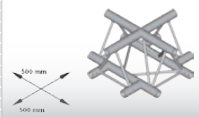
4 Weg Kreuzstück Gewicht 5,7 kg
