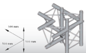
4 Weg Eckstück 90° / links Gewicht 6,5 kg
