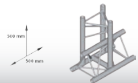
3 Weg T-Stück vertical - Spitze unten Gewicht 5,3 kg
