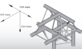
4 Weg T-Stück vertical - Spitze oben Gewicht 6,1 kg
