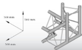
3 Weg Eckstück 90° - Spitze oben links Gewicht 5,1 kg
