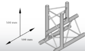
3 Weg T-Stück - vertical Gewicht 5,5 kg
