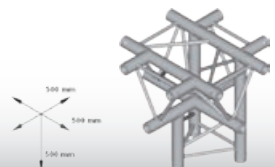
5 Weg Kreuzstück - Spitze unten Gewicht 7,2 kg
