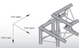
3 Weg Eckstück 90° - Spitze oben rechts Gewicht 5,1 kg
