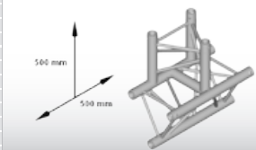
3 Weg T-Stück - horizontal Gewicht 4,6 kg
