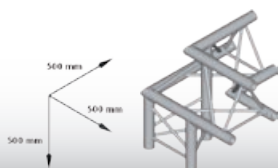
3 Weg Eckstück 90° - Spitze oben links Gewicht 5,1 kg
