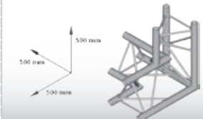
3 Weg Eckstück 90° - Spitze oben rechts Gewicht 5,1 kg
