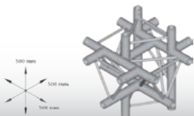
6 Weg T-Stück Gewicht 9,8 kg
