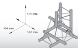
4 Weg T-Stück vertical - Spitze unten Gewicht 6,1 kg
