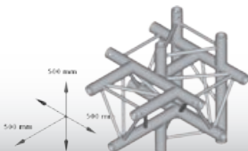
5 Weg T-Stück Gewicht 7,6 kg
