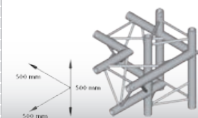
4 Weg Eckstück 90° / rechts Gewicht 6,5 kg
